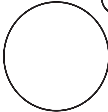
Jupiter
